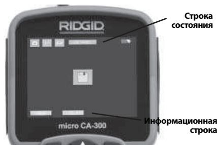
Рис. 13 - Рабочий экран
